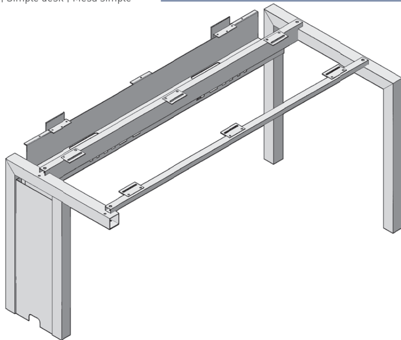
CORTE ESQUEMÁTICO | SCHEMATIC SECTION | CORTE ESQUEMÁTICO Mesa dupla com trilho | Double desk with rail | Mesa doble con riel
